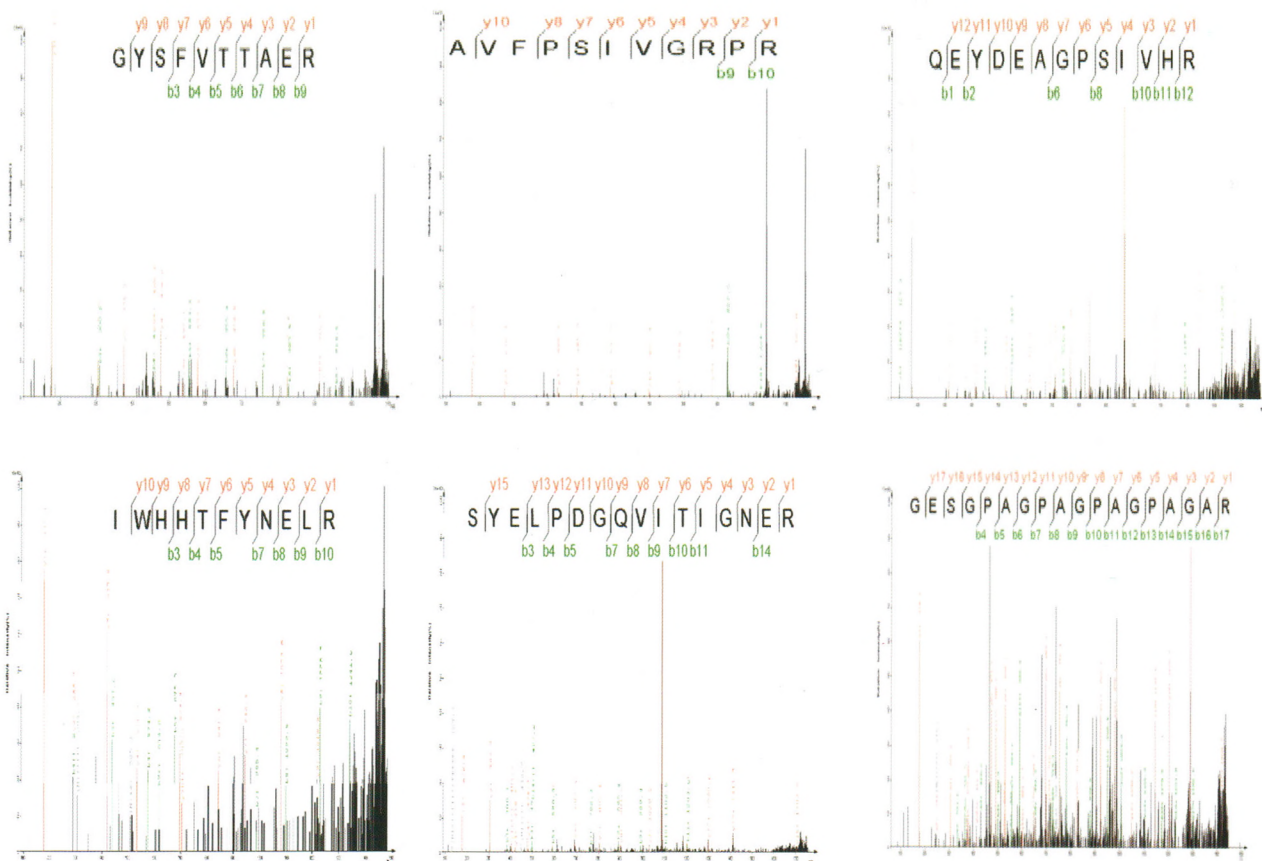
图 3 母离子碎片串联质谱图 (其中 A,B,C,D,E 为图 2 中标记的母离子匹配序列,F 为图 3 中标记的母离子匹配序列)
