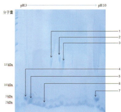
图 1 蕲蛇乙醇提取物中多肽的双向凝胶电泳图谱(1~7 为切取进行质谱鉴定的胶点)
