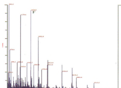
图 4 3号胶点一级质谱图 (F 为成功鉴定的肽段母离子峰)
