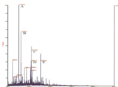
图 2 2号胶点一级质谱图 (A,B,C,D,E 为成功鉴定的肽段母离子峰)
