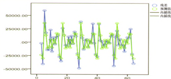
图4 残差拟合值
