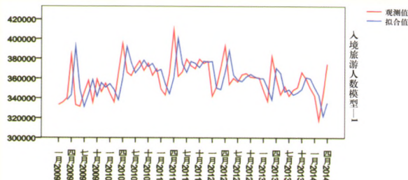
图3 拟合结果
