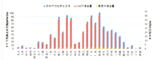
图2 各地区多年平均地表水资源量和污染物COD、氨氮的水环境容量
