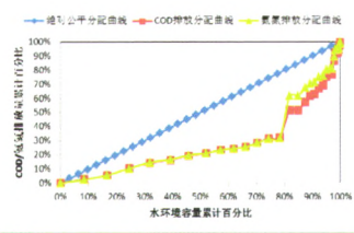
图3 水环境容量—COD/氨氮排放量的洛伦茨曲线
