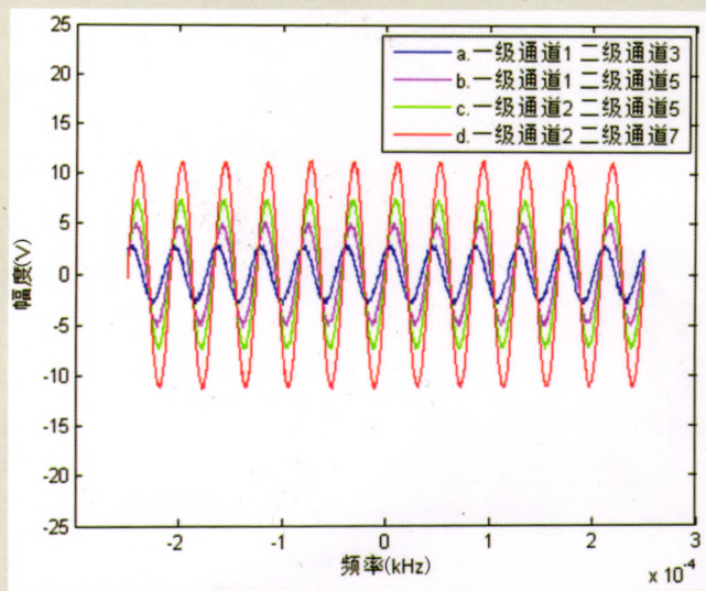
图9 程控功率放大功能部分档位测试结果
