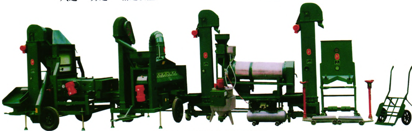
5XJG-3.0 型谷物种子加工机组
